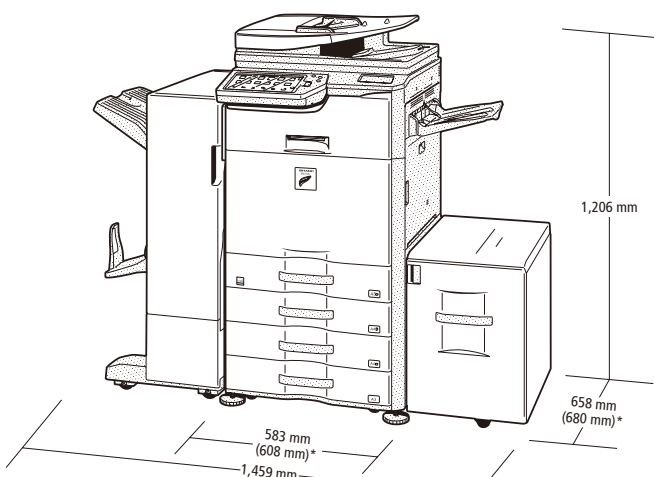
* MX-3610N dimensions
